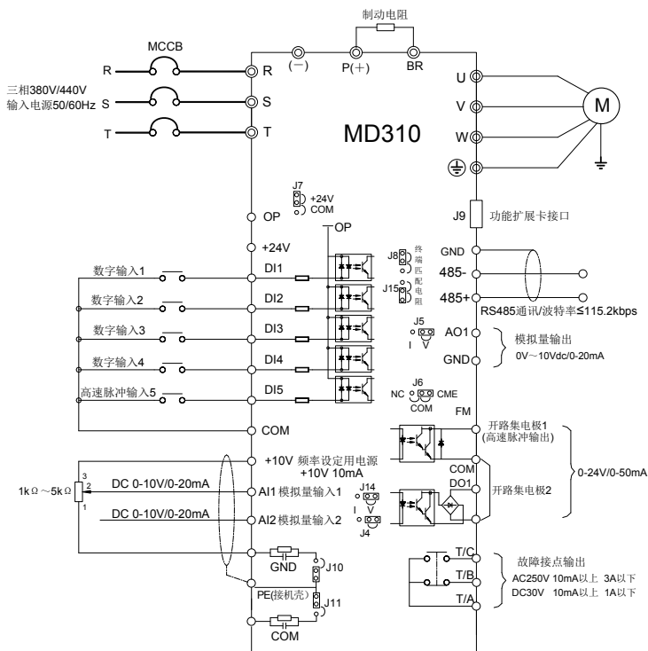
图 3-19 MD310 系列变频器接线示意图
