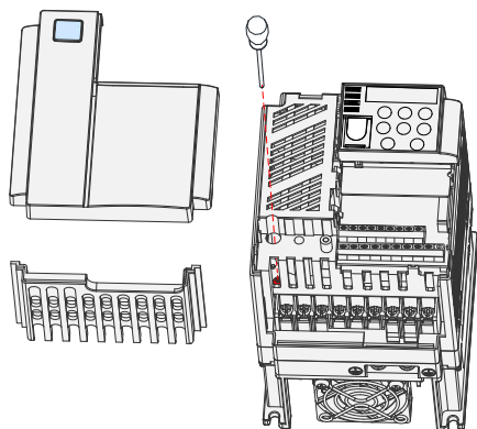
图 7-10 MD310T0.4B、MD310T0.7B、MD310T1.5B、MD310T2.2B 压敏电阻（VAR）和安规电容共同对 PE 连接的螺钉位置示意图
