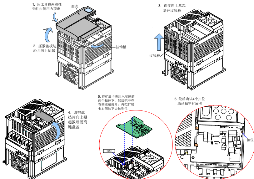
图 B-2 MD310-IO1 扩展卡安装步骤
