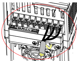
图 7-6 屏蔽电缆接地示意图
