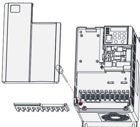
图 7-11 MD310T3.7B、MD310T5.5B 压敏电阻（VAR）和安规电容共同对 PE 连接的螺钉位置示意图
