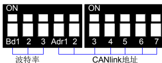
图 C-3 MD310-CANL拨码开关
