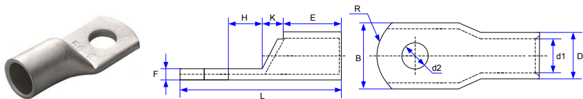
图 3-10 GTNR 系列圆型线耳外观及尺寸图（推荐）
