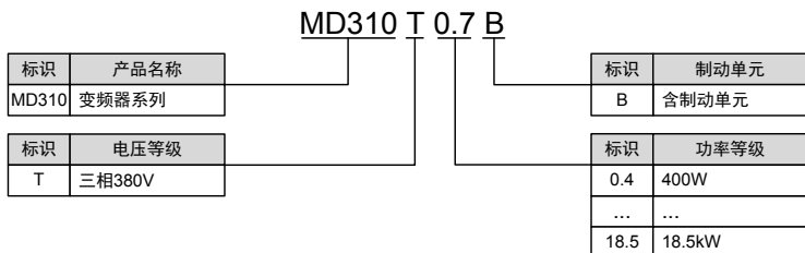
图 2-1 铭牌信息与产品命名
