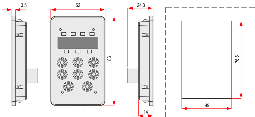
图 D-3 MD310-KEY1 外引键盘安装尺寸图（单位：mm）
