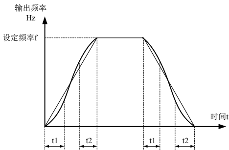
图 6-17 静态 S 曲线加减速示意图
