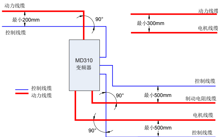
图 7-7 电缆布线图
