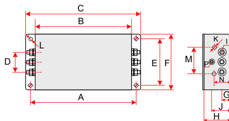
图 7-3 扼流滤波器 DL-25EBK5/ DL-35EBK5/ DL-50EBK5 尺寸图
