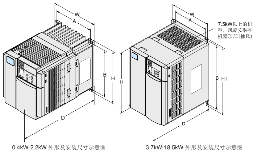
图 2-3 MD310 系列外型尺寸及安装尺寸示意图
