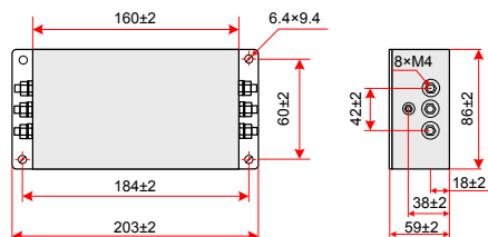
图 7-2 扼流滤波器 DL-5EBK5 尺寸图 (单位: mm)
