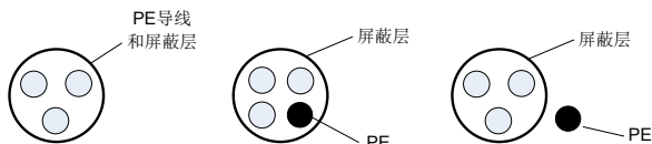
图 7-4 屏蔽电缆侧面示意图
