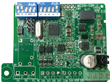
图 C-1 CANlink 通信扩展卡 MD310-CANL
