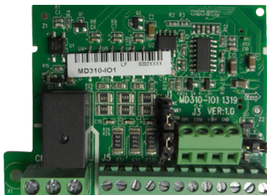
图 B-1 多功能 IO 扩展卡
