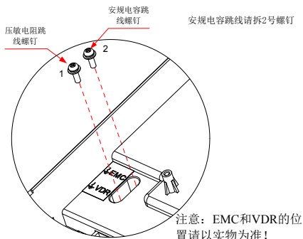
图 7-9 MD310T7.5B、MD310T11B、MD310T15B、MD310T18.5B 安规电容跳线位置及断开方法
