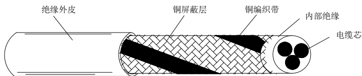
图 7-5 屏蔽层的编织密度
