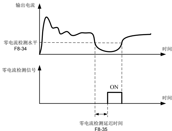
图 6-27 零电流检测示意图
