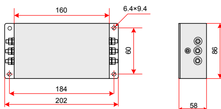
图 7-3 扼流滤波器 DL-10EBK5/ DL-16EBK5 尺寸图 (单位: mm)
