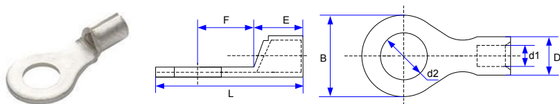
图 3-11 TNR 系列圆型线耳外观及尺寸图（推荐）
